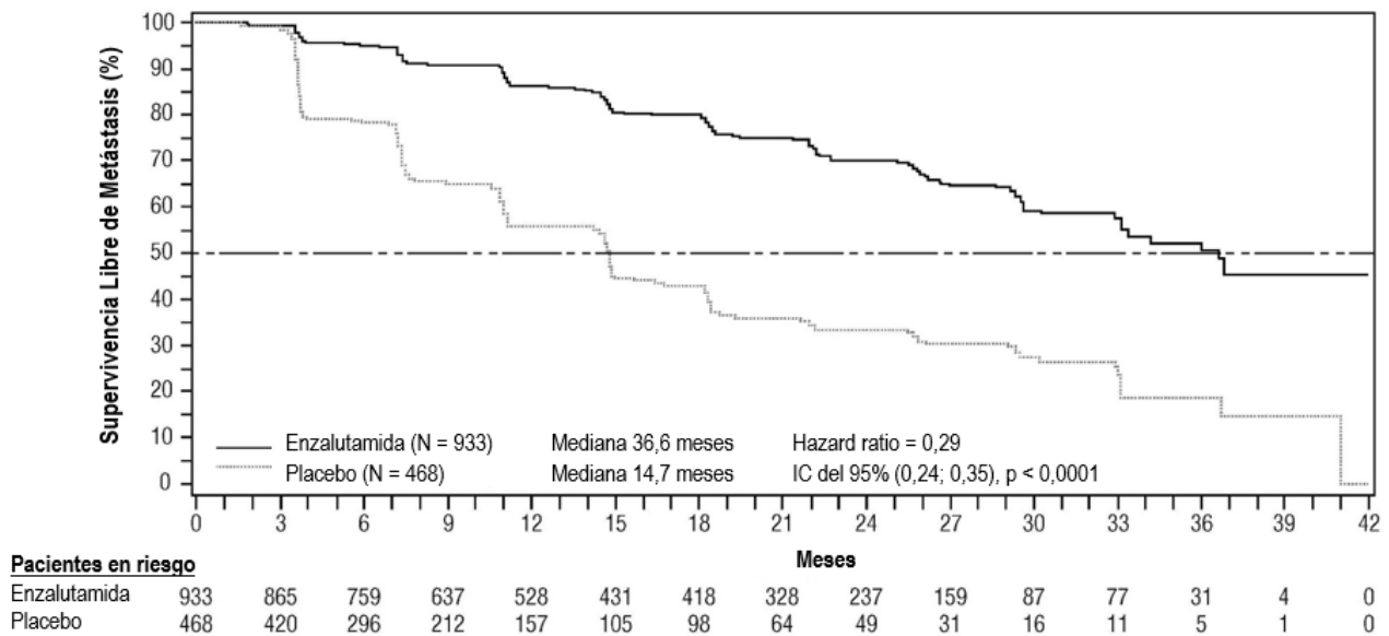
Figura 1: Curvas de Kaplan-Meier de supervivencia libre de metástasis en el ensayo PROSPER (análisis por intención de tratar)
