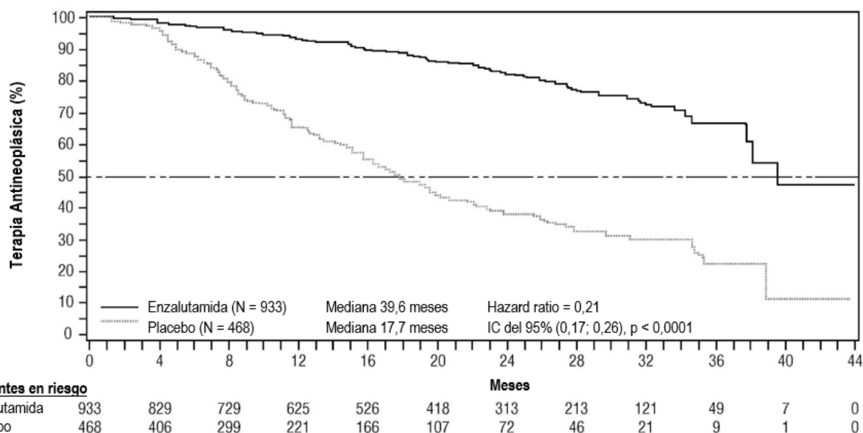
Figura 2: Curvas de Kaplan-Meier del tiempo hasta el primer uso de una nueva terapia antineoplásica en el ensayo PROSPER (análisis por intención de tratar)
