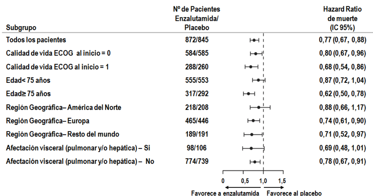
Figura 5: Análisis de supervivencia global actualizado por subgrupos. Hazard ratio e intervalo de confianza del 95% en el ensayo PREVAIL (análisis por intención de tratar)
