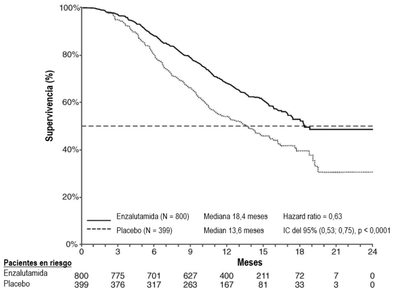
Figura 7: Curvas de Kaplan-Meier de supervivencia global en el ensayo AFFIRM (análisis por intención de tratar)
