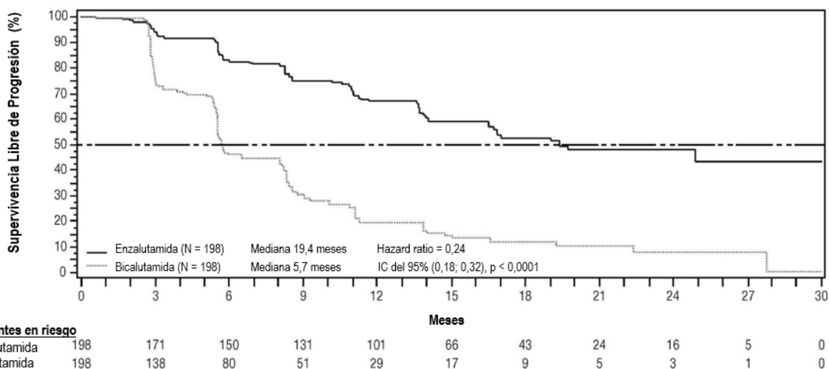
Figura 3: Curvas de Kaplan-Meier de supervivencia libre de progresión en el ensayo STRIVE (análisis por intención de tratar)
